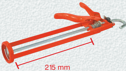
Nr. 2179/SX Kartuschen-Pistole Best Nr. 2179/SX Skelett aus Metall Profiausführung
