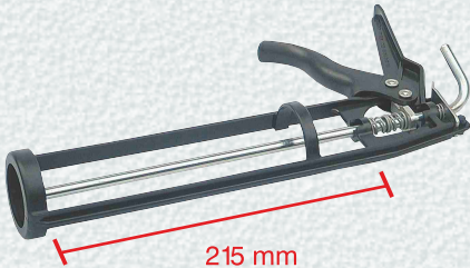
Nr. 2179/S Kartuschen-Pistole Best Nr. 2179/S Skelett aus Kunststoff, daher leicht und warm im Griff stabile Ausführung
