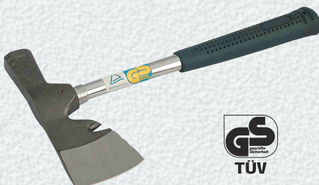
Nr. 2354/P Gipserbeil
